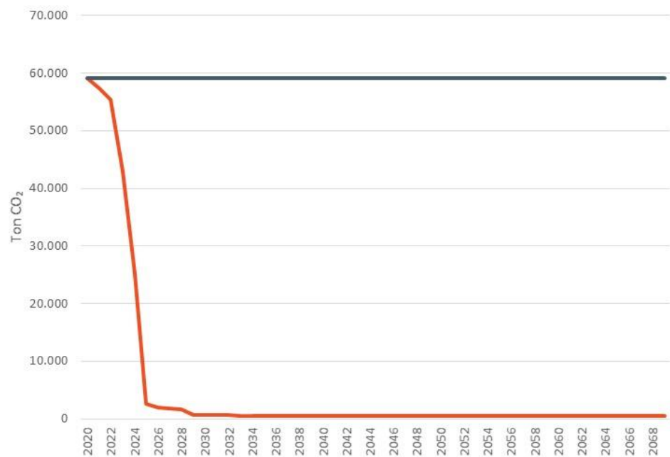
Figur 6-12 CO 2 -udledning for scenarie 3 og baseline, ton frem mod 2070
