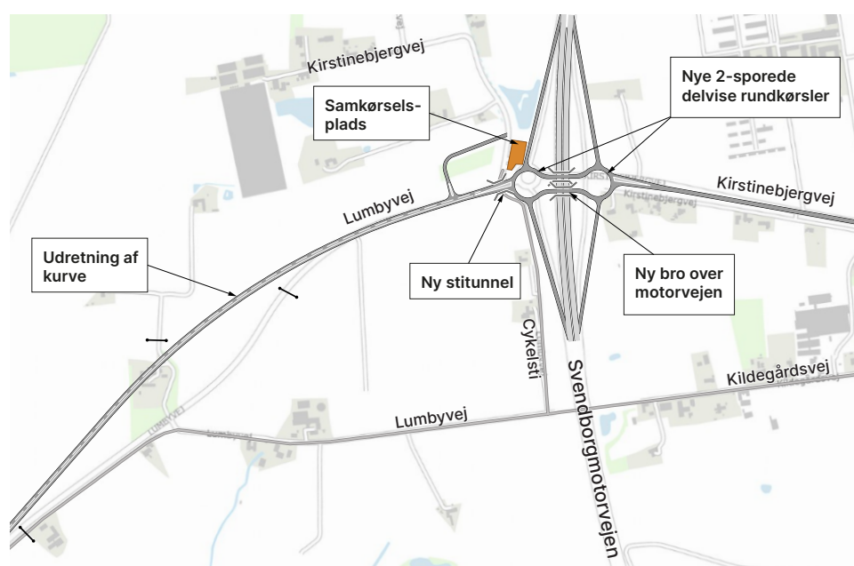
Figur 4.13 Ombygning af tilslutningsanlæg 11 ved Årslø.
