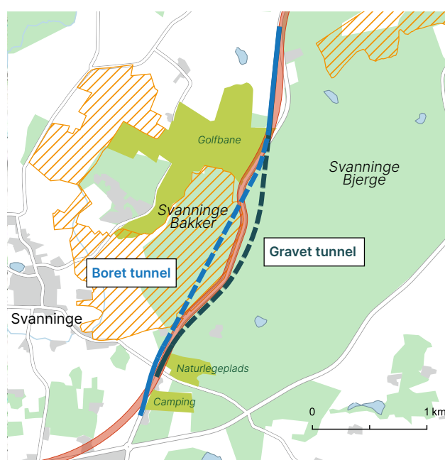
Figur 4.11 Undersøgte tunnelloesninger ved Svanning Bakker.
