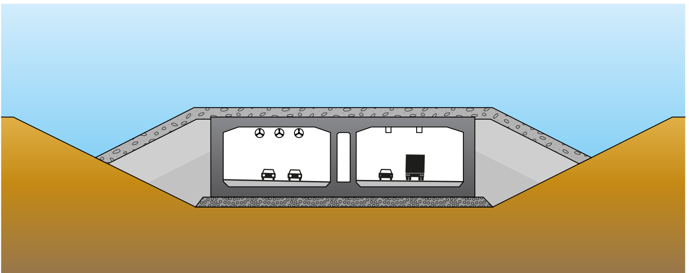
Normaltværsnit i Egholmtunnelen, udgravning og tilfyldning for sænketunnel
